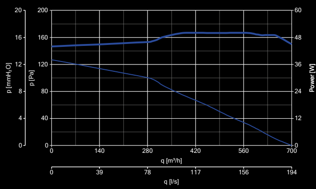
LINEO 200 Q - LINEO 200 Q T - VELOCITÀ MIN
