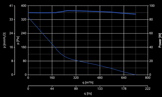
LINEO 250 Q - LINEO 250 Q T - VELOCITÀ MIN
