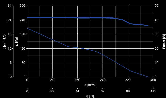
LINEO 160 - LINEO 160 T - VELOCITÀ MIN
