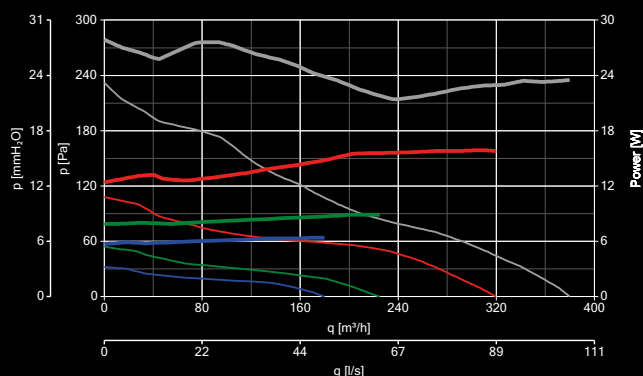
LINEO 125 QUIET ES
