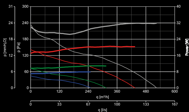
LINEO 160 QUIET ES
