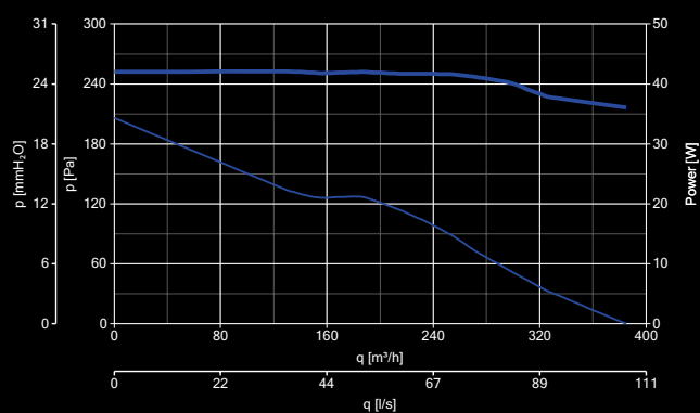
LINEO 150 - LINEO 150 T - VELOCITÀ MIN
