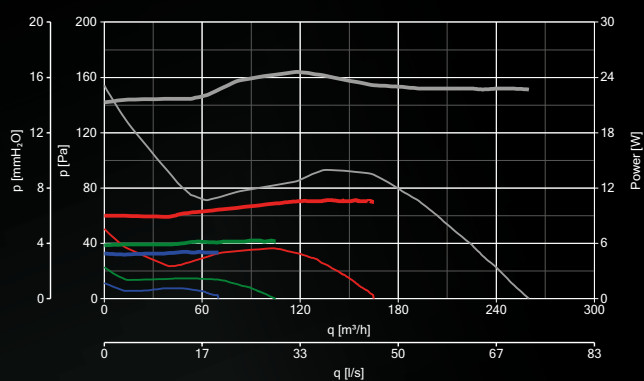
LINEO 100 Q ES
